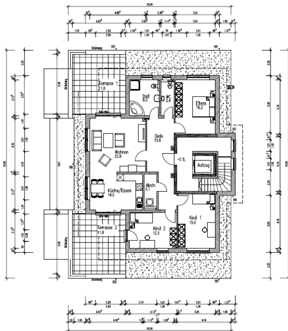
Dachgeschoss
